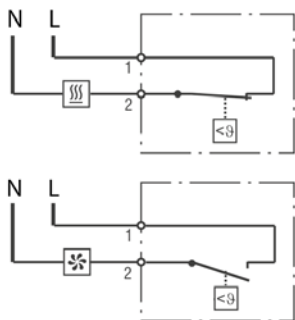
Схемы подключения
